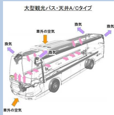
○外気導入固定運転による 車内換気(一部車両のみ)
